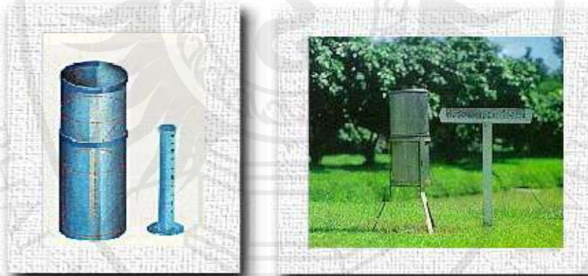
รูปที่ 2.8 ถังวัดน้ำฝนแบบแก้วตวง (RAIN GAUGE)
