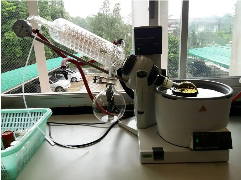
ภาพภาคผนวกที่ 1 เครื่องระเหยสุญญากาศ (rotary evaporator)
