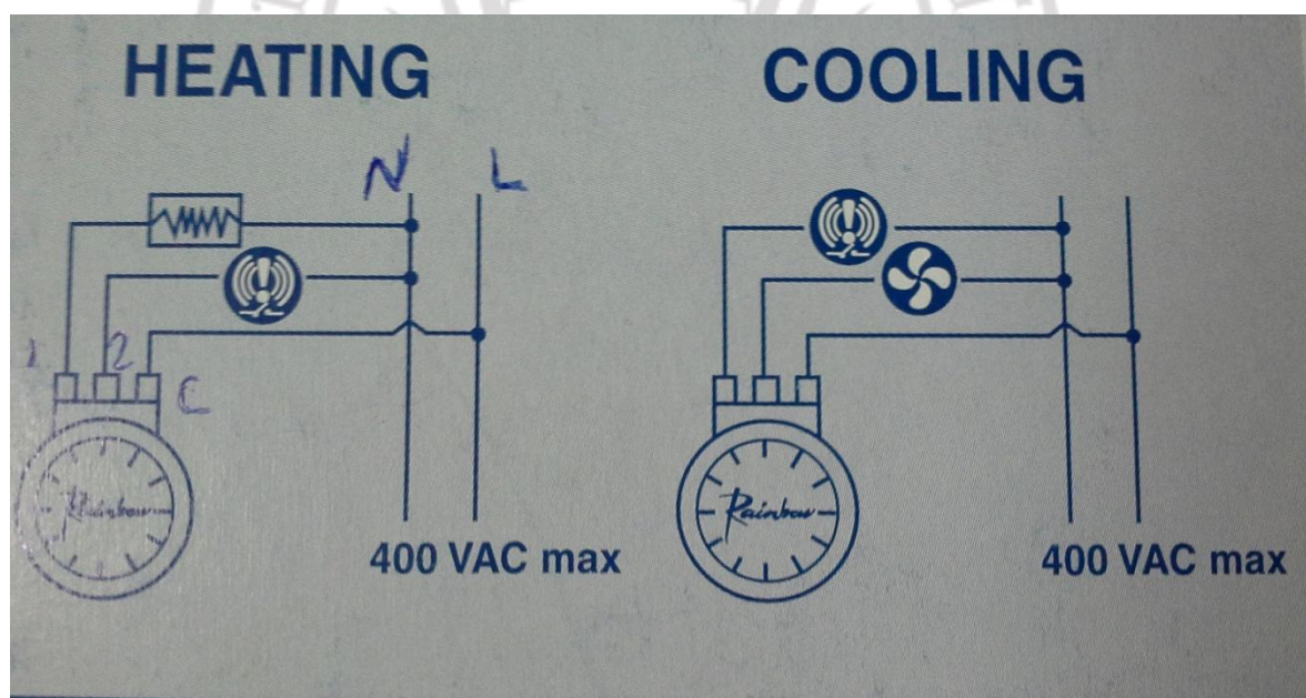
ภาพที่ ก.4 ลักษณะการต่อวงจรไฟฟ้าของชุด Thermostat ยี่ห้อ Rainbow
