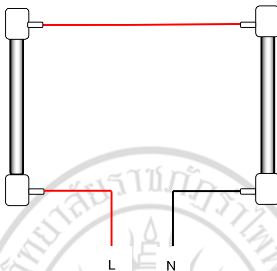
ภาพที่ ก.1 ลักษณะการต่อวงจรไฟฟ้าของชุดฮีตเตอร์อินฟราเรด (ต่อแบบอนุกรม)
