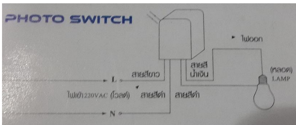
ภาพที่ ก.3 ลักษณะการต่อวงจรไฟฟ้าของชุด Photo Switch ยี่ห้อ GATA
