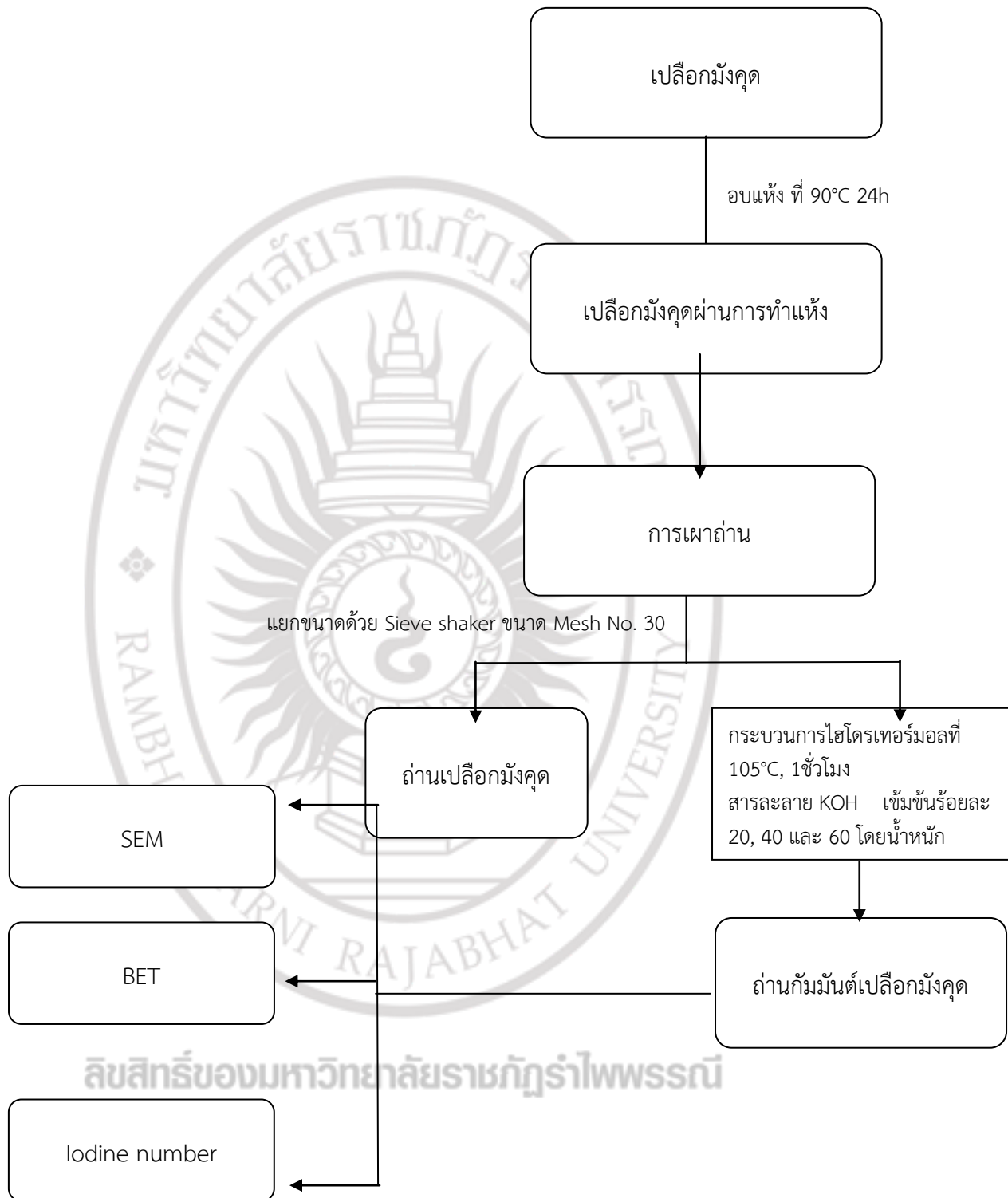
ภาพที่ ก.1 แผนผังแสดงการเตรียมถ่านกัมมันต์จากเปลือกมันาคุดเหลือทิ้งในกระบวนการแปรรูปของวิสาหกิจชุมชนคลองน้ำเค็มทันใจ ด้วยเทคนิคไฮโดรเทอร์มอล
